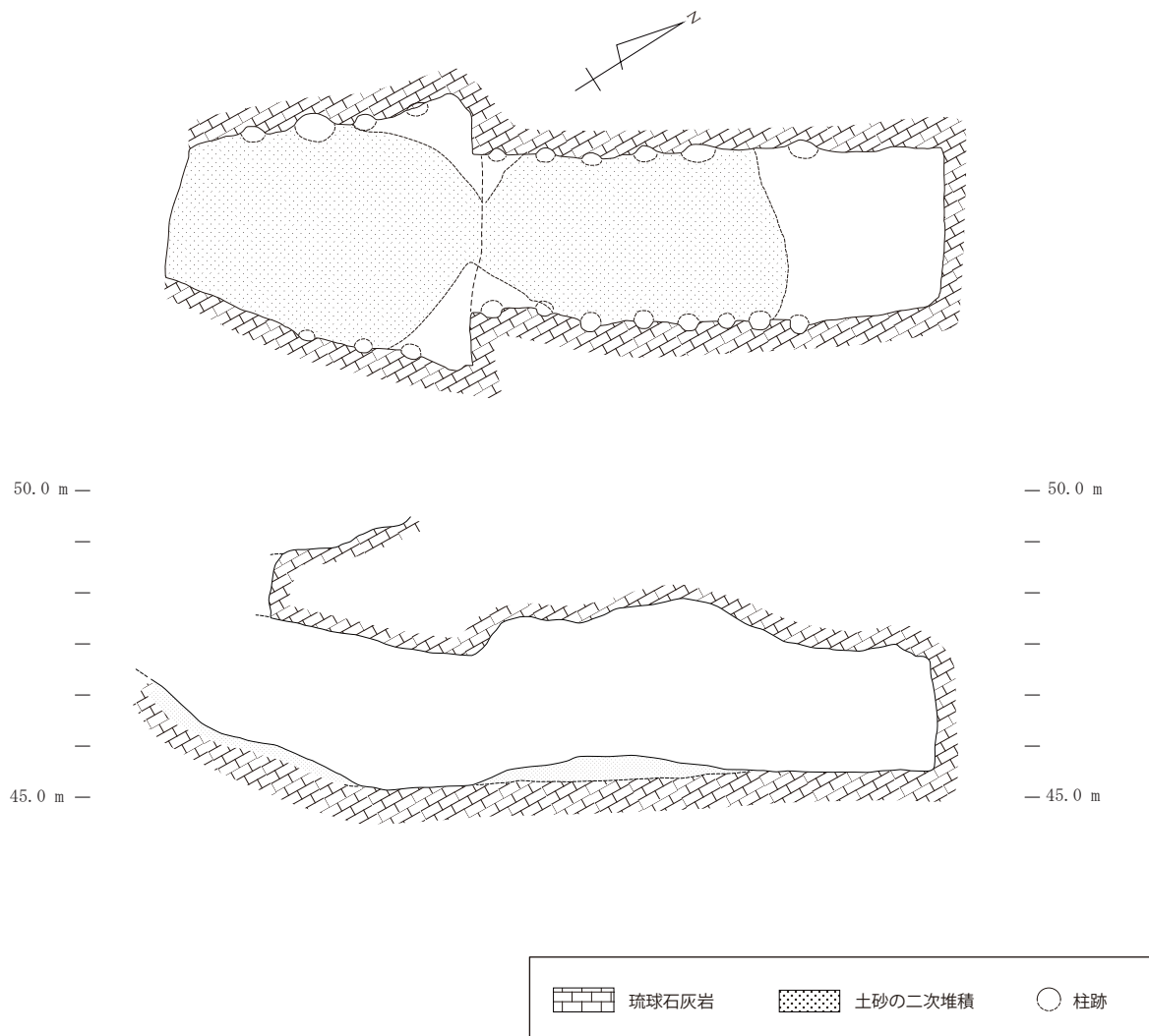
第10図 壕3平面図・断面図 (S=1/150)
