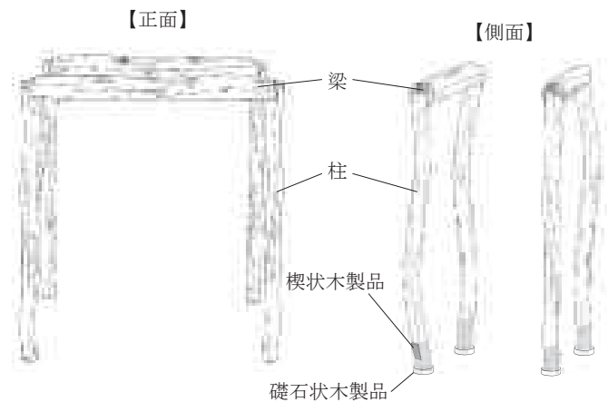
第 7 図 壕内の坑木利用模式図（宮古島市教育委員会 2015）
